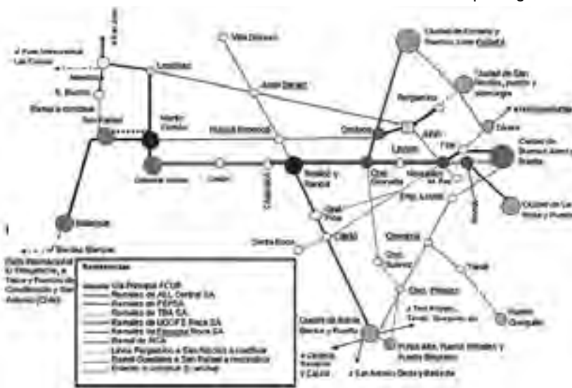
Detalle del Esquema Ferroviario principal del Proyecto elaborado por el "Consorcio Ferroviario Unión Pacífico". Ver más en: http://www.unionpacifico.com.ar
